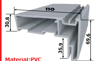
İ-757-B
