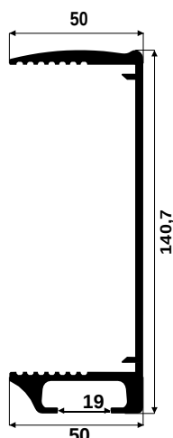
I-410-11
