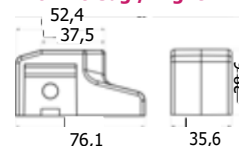
I-761-10 Sağ / Right
