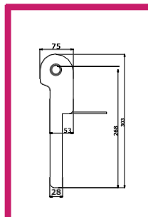
I-SKA-18-01RP Izq/left
