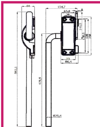
Dibujo Técnico / Drawing
