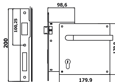
Dibujo Técnico / Drawing
