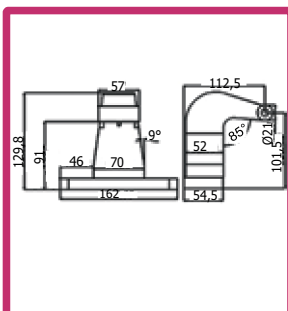
I-SKA-06
